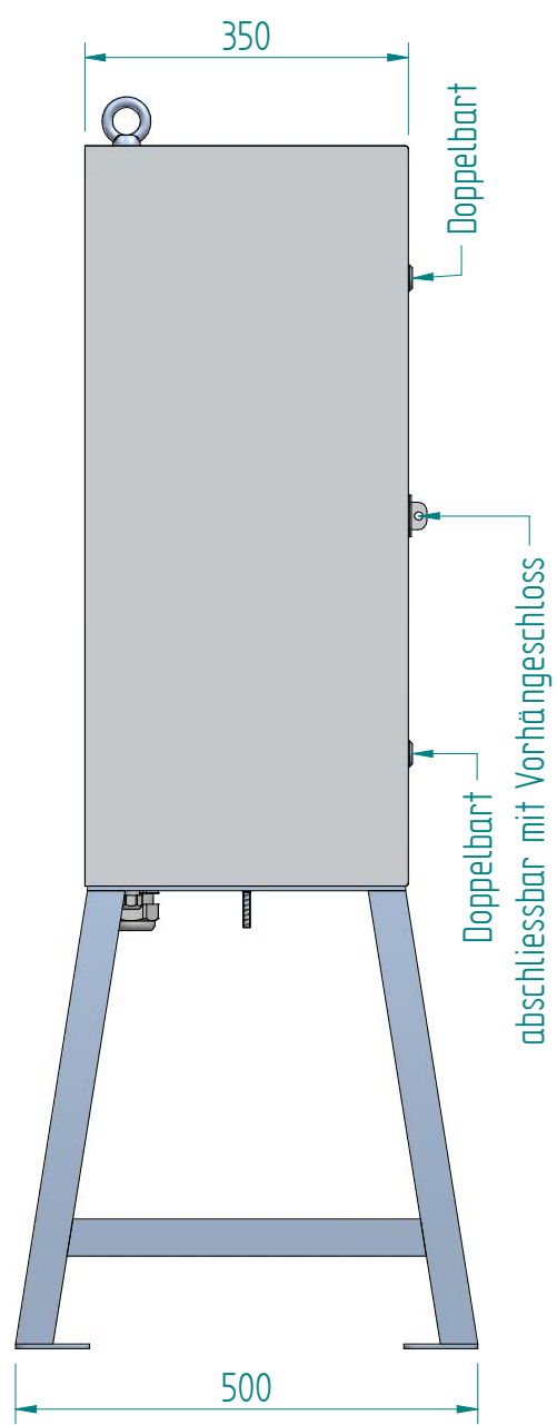
Schema Art.Nr. 231124
