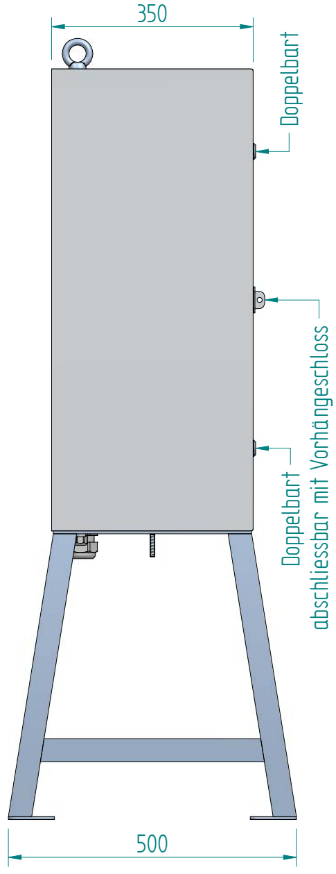
Schema Art.Nr. 231120
